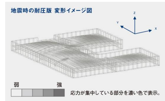
構造計算
