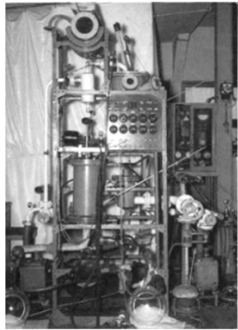
創業時の製造装置
