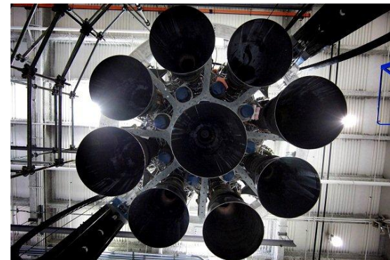
Falcon9ロケットのエンジン
